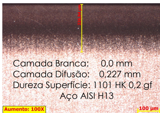
Camada nitretada em aço AISI H13 para aplicações industriais, por exemplo, Injeção de Plástico; Forjamento a Quente (sem / com camada branca);
