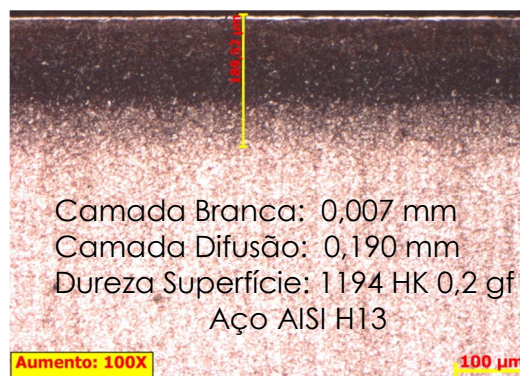
Camada nitretada em aço AISI H13 para aplicações industriais, por exemplo, Injeção de Plástico; Forjamento a Quente (sem / com camada branca);
