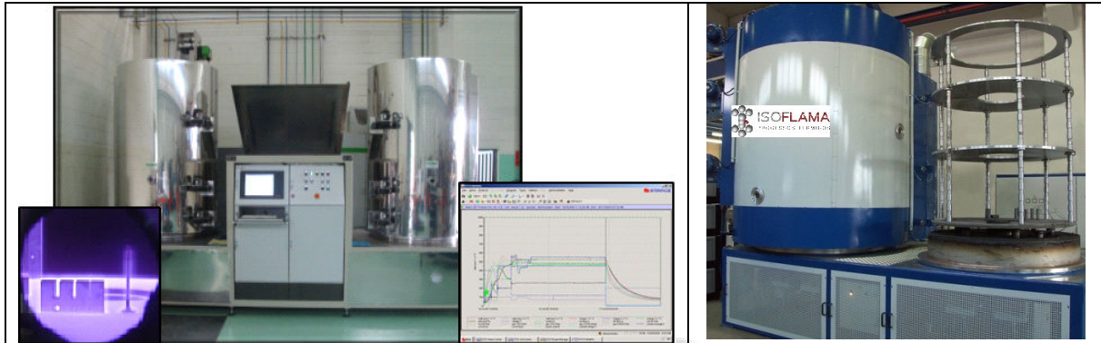
Figura 1 – Fornos de nitretação a plasma e gráfico dos parâmetros de nitretação a plasma
