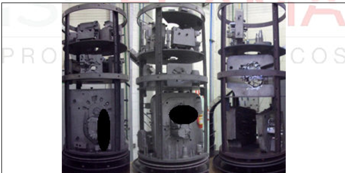
Figura 3 – Moldes injeção alumínio montados no forno de nitretação plasma
