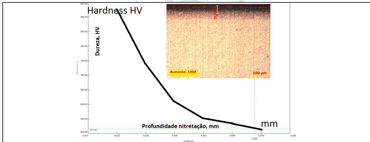
Figura 2 – Curva de microdureza (NHT) na camada nitretada
