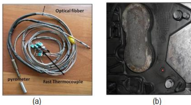
Fig. 1. (a) Sonda de transferencia de calor y (b) posición de la sonda en el molde.
