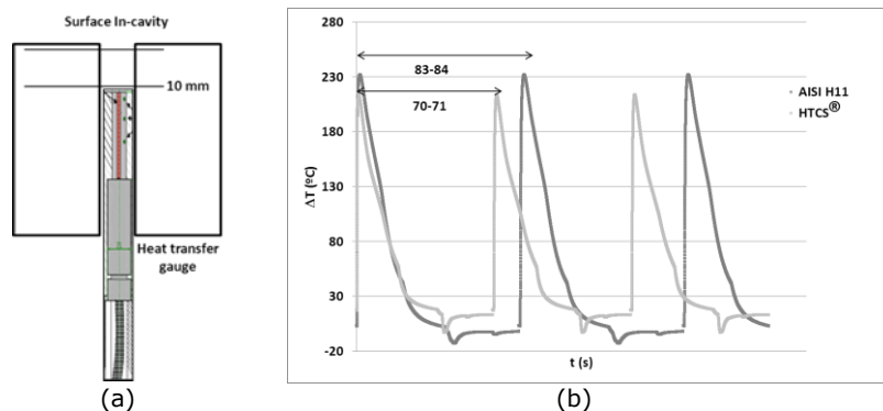
Fig. 8. (a) posición de la sonda de temperatura en el molde y (b) perfiles de temperatura experimentales cerca de la superficie del molde y a 10 mm durante tres ciclos de inyección consecutivos para AISI H11 (gris oscuro) y HTCS® (gris claro).
