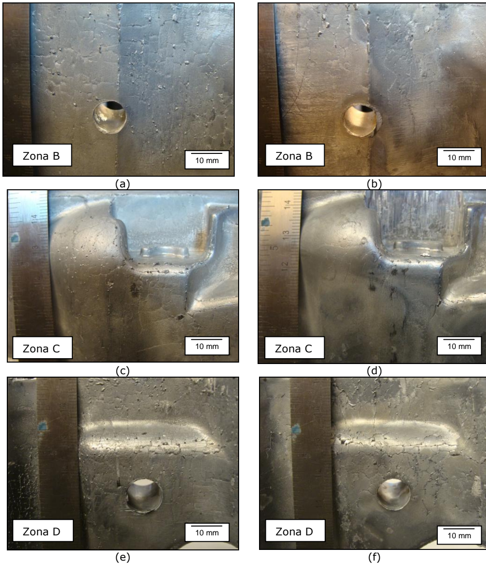
Fig. 5. Grietas de fatiga térmica de la superficie del componente inyectado después de 75.000 ciclos. (a, c y e) corresponden al molde de AISI H11 y (b, d y f) al molde de HTCS®.
