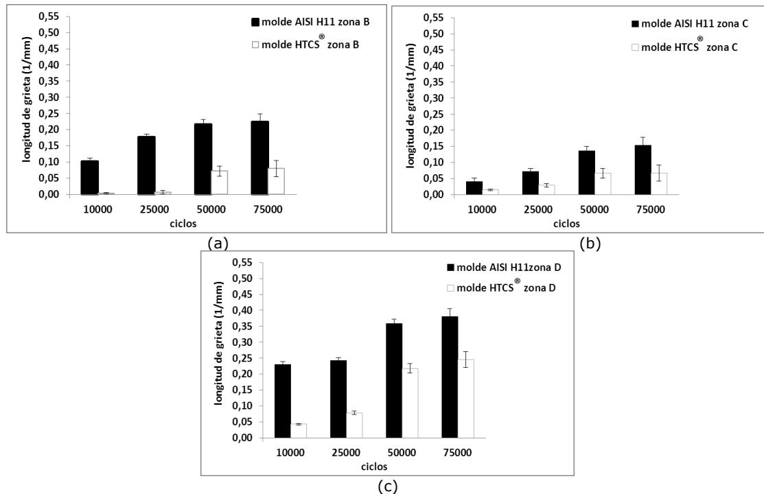
Fig. 7. Longitud de grieta ( L_{crack} ) en las zonas B, C y D para los dos moldes AISI H11 y HTCS®.
