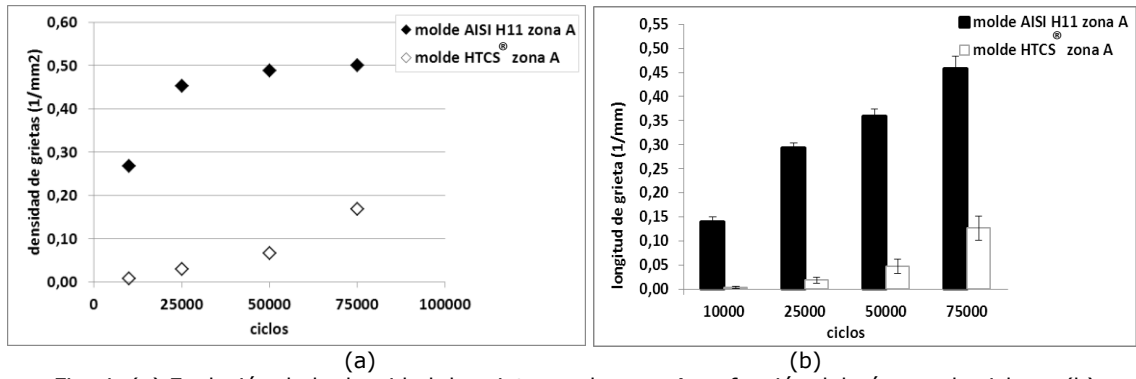
Fig. 4. (a) Evolución de la densidad de grietas en la zona A en función del número de ciclos y (b) evolución de la longitud de grieta ( L_{crack} ) en la zona A en función del número de ciclos.
