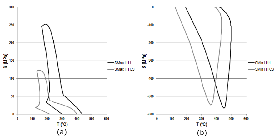
Fig. 10. Esfuerzos principales en función de la temperatura correspondientes al punto de la superficie. Ciclo en estado estacionario. ((a) máximo, (b) mínimo)
