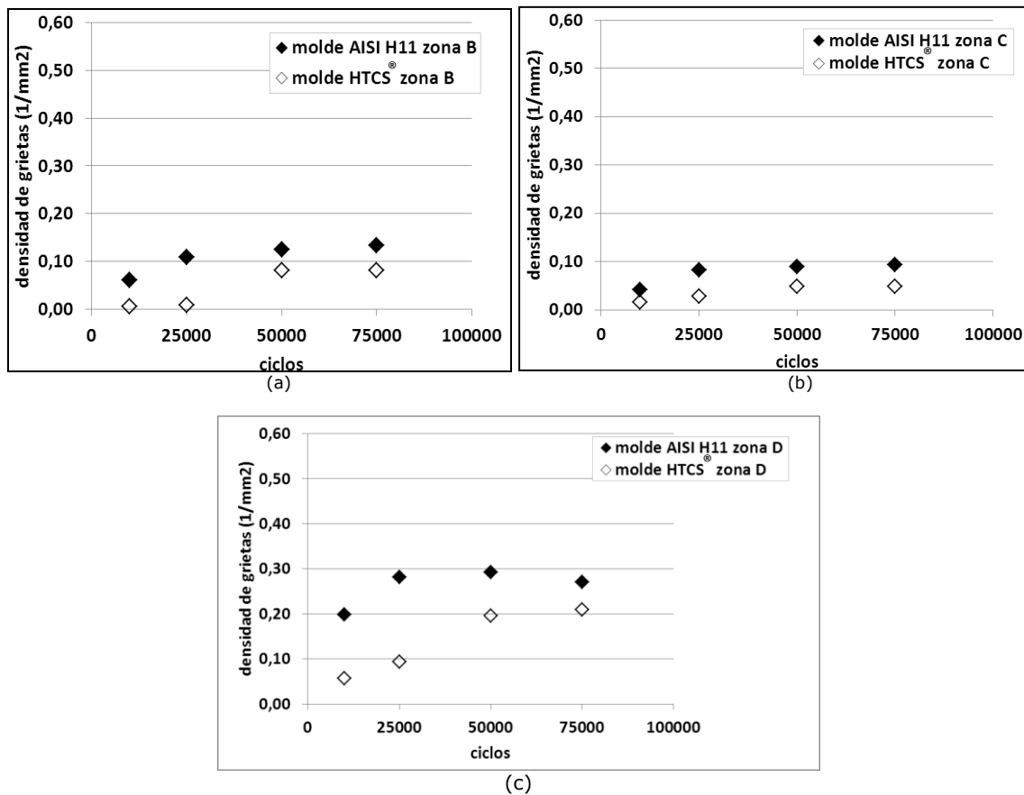
Fig. 6. Densidad de grietas de (a) zona B, (b) zona C y (c) zona D a diferentes ciclos para los dos moldes.
