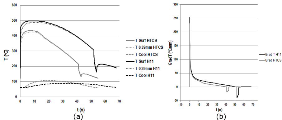
Fig. 9. (a) Evolución de la temperatura para un ciclo en estado estacionario correspondiente a moldes de HTCS® y de AISI H11 y (b) evolución temporal del gradiente de temperatura entre la superficie y el punto a 0.39mm de profundidad correspondiente a un ciclo en estado estacionario.
