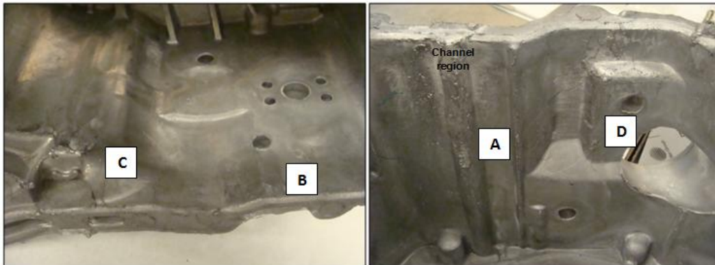
Fig. 2. Las cuatro zonas analizadas del componente inyectado.
